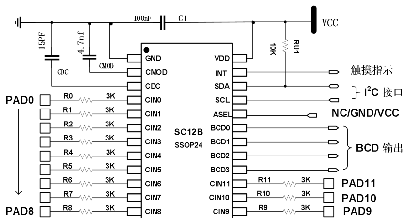
图 3-1 : 应用电路
